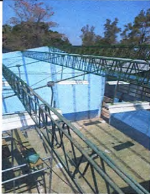
Foto 1: Estructura de Techo Limpia
